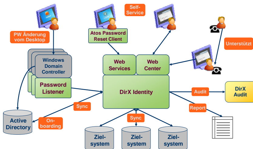
Abb. 3 - DirX Identity Passwortmanagement Architektur
